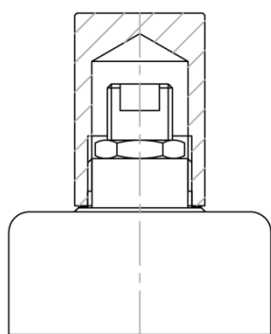
Capuz roscado Tipo "A"
