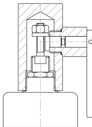
Capuz roscado Tipo "E"
