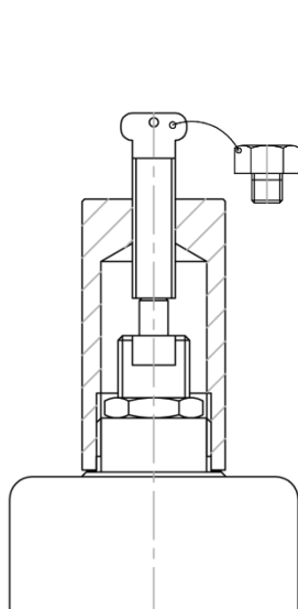
Capuz roscado Tipo "B" Com trava para teste
