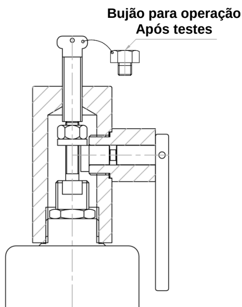
Capuz roscado Tipo "F" Com trava para teste
