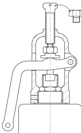
Capuz parafusado Tipo "D" Com trava para teste
