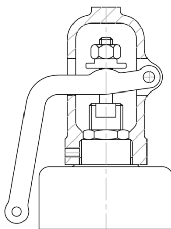
Capuz parafusado Tipo "C"
